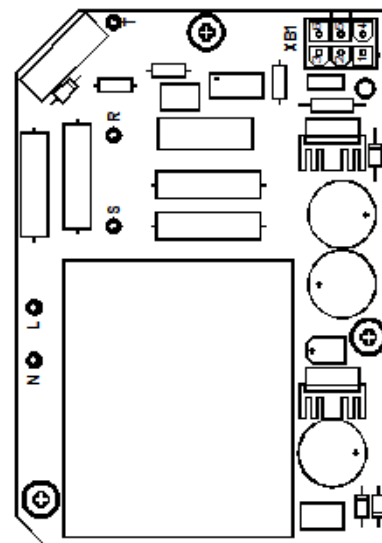
Bild 2: Spannungsversorgung
