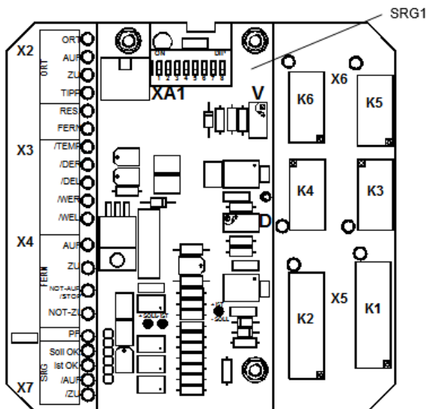
Bild 1: Logikplatine mit Stellungsregler SRG
